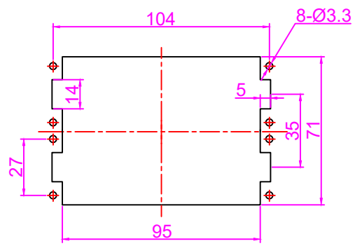
面板开孔图 Panel cut
